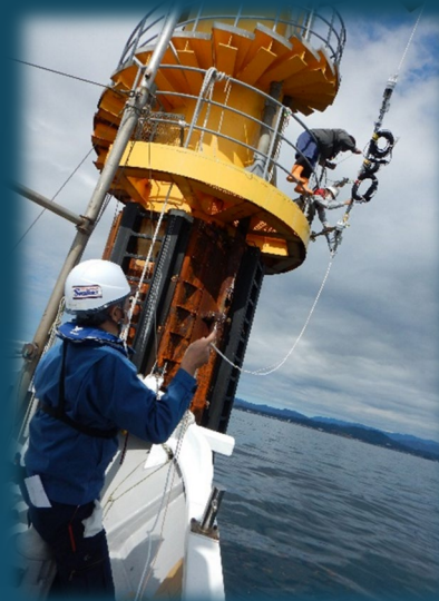
観測塔への計測機器設置作業
