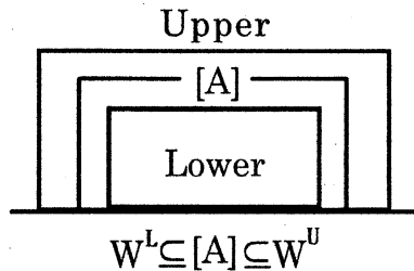
図 1: 区間一対比較値の上界・下界近似
