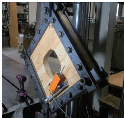
図1：開口を持つ CLT 要素のせん断実験
