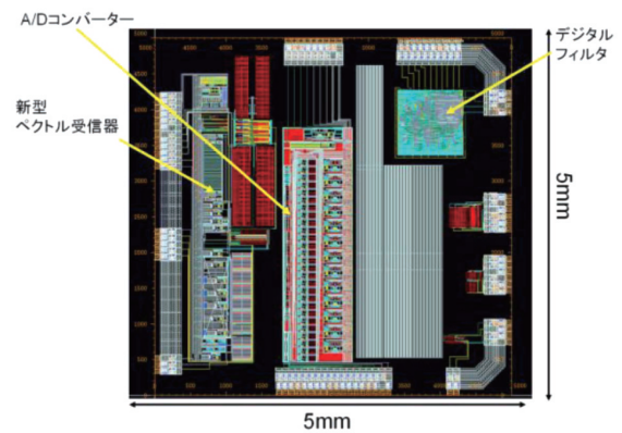
図1：アナログとデジタルを混載した初めてのプラズマ波動観測器チップのチップ内レイアウト
