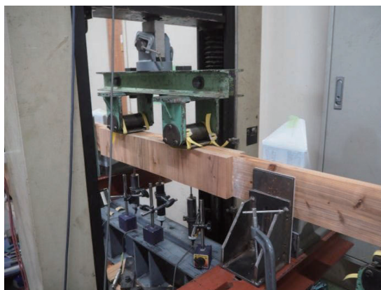
図2：直交部材による補強効果確認
