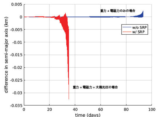
図1：宇宙デブリ帯電による軌道長半径の時間変化
