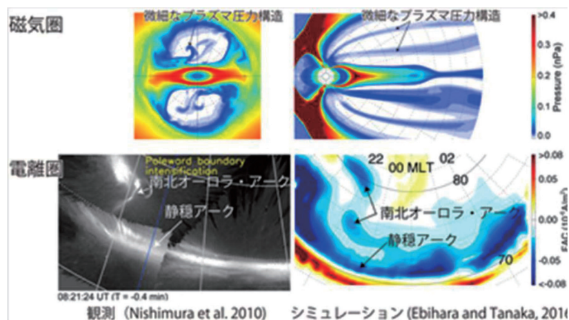
図3：オーロラ・アークのシミュレーション
