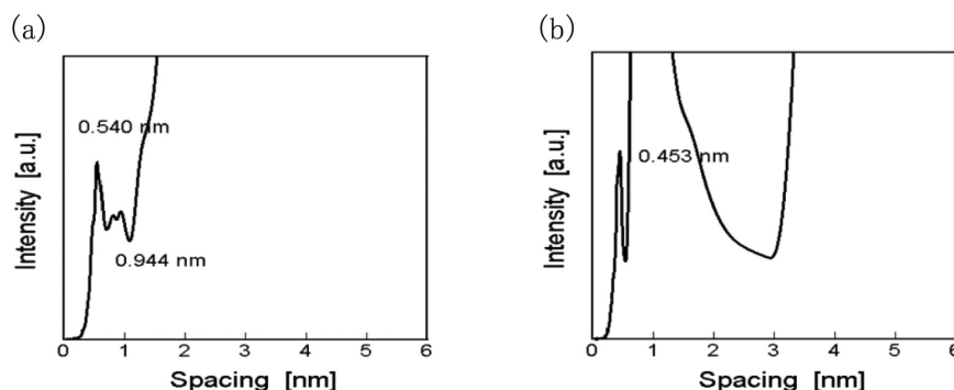
図4：2D-FFTによって得られた空隙分布 (a)AO照射前、(b)AO照射後
