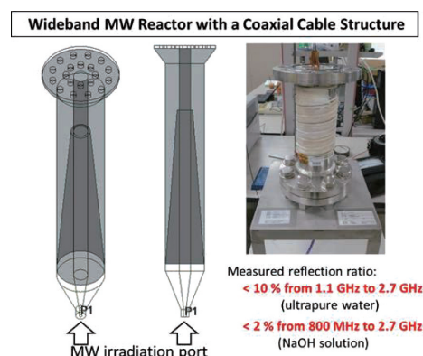
図7：化学反应用マイクロ波加熱容器の研究開発
