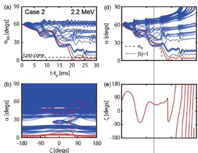
図2：EMIC波とのサイクロトロン共鳴散乱によってロスコーンに降下する粒子の軌跡（赤）
