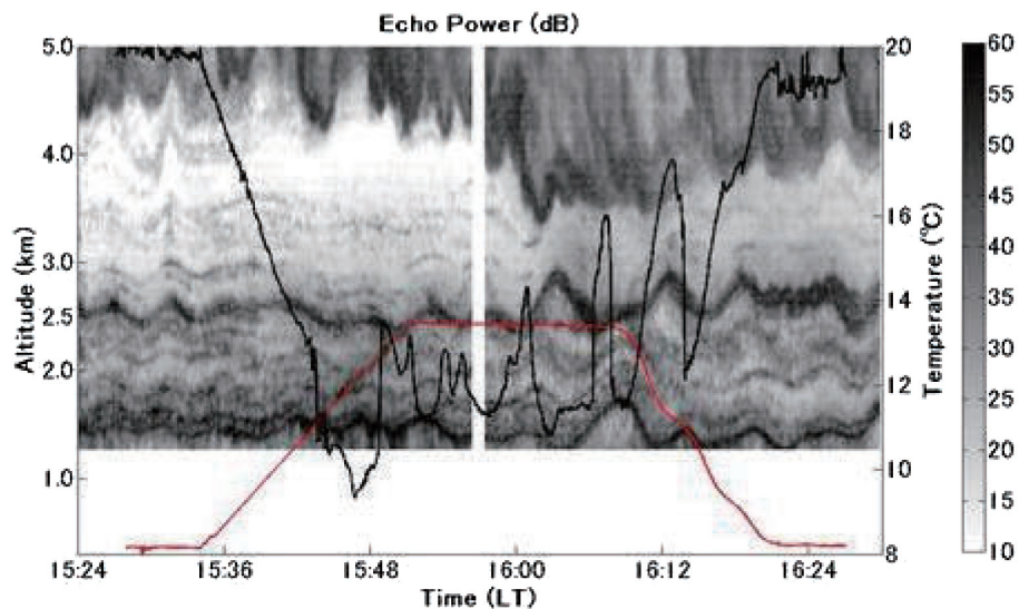
図1：2015年6月9日15時24分～16時30分に MU レーダー天頂ビームのレンジイメージングモードで得られたエコー強度の時間高度変化と UAV の飛行高度（赤線）および UAV 搭載センサーで得られた気温（黒線）の時間変化。
