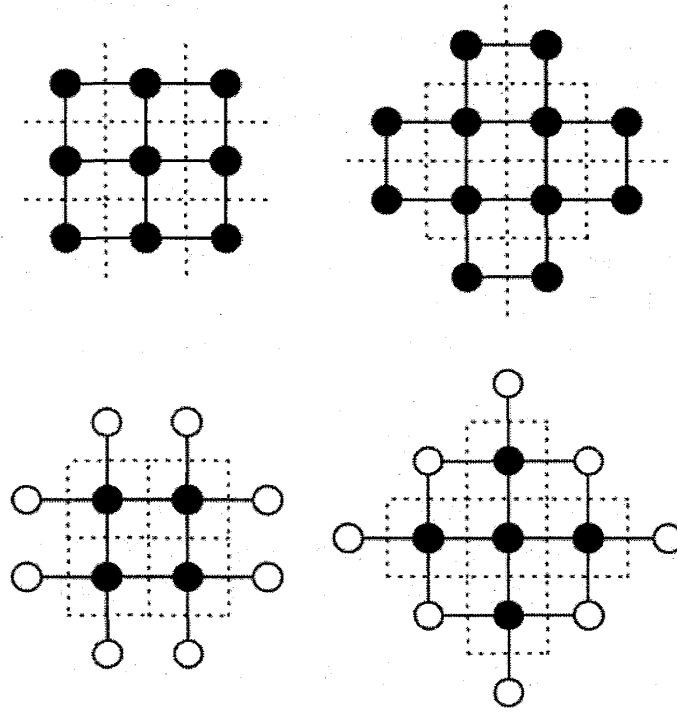
図 6: 双対変換による格子の変化の 2 例. 上側が双対変換前の格子であり, 下側がそれらの双対変換後の格子である. 黒丸で表されたスピンの和を取る部分であり, 白丸のスピンの場合には上向きで固定された条件を課す.
