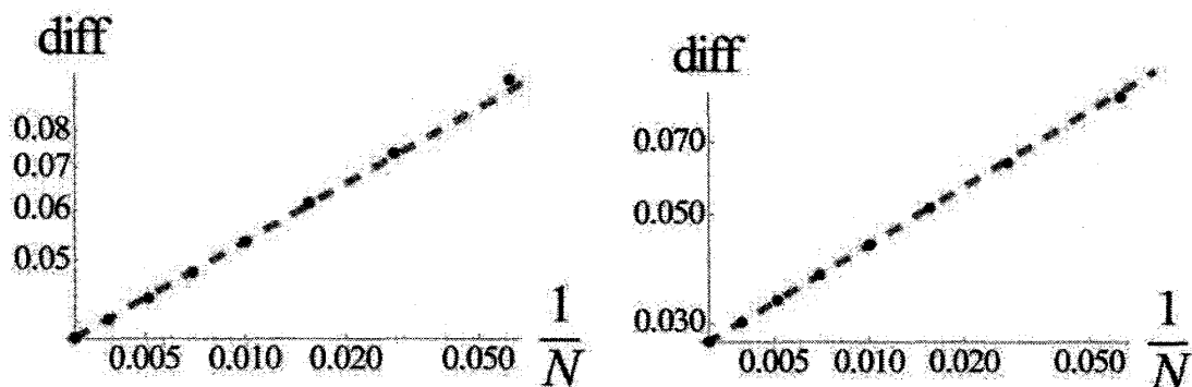
図 31: 正方格子の場合に利用する系統的なユニット.
