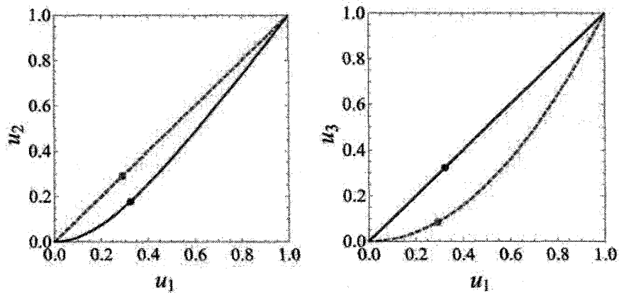
図 14: 西森線上のレプリカ数 2 における \pm J Ising 模型の相対 Boltzmann 因子の振る舞い. ランダムさが ない場合と同様に双対変換前のものと後のものでは完全に一致する.
