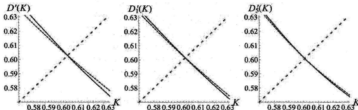
図 26: レプリカ数 3 に対する有効 \pm J Ising 模型における温度の変換関数 D_r'(K) とその逆関数 D_r'^{-1}(K) の振る舞い. 左から繰り込みを行わない場合 ( D_r'(K) ), 1 回繰り込みを行った場合 ( D_1'(K) ), 5 回繰り込みを行った場合 ( D_5'(K) ).
