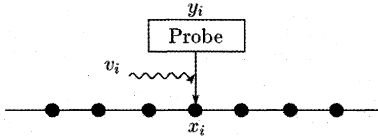
図 35: 1次元鎖状におかれた情報の系列. デバイスで x_i をひとつずつ読み出していき, 右方向にスライドしていく.
