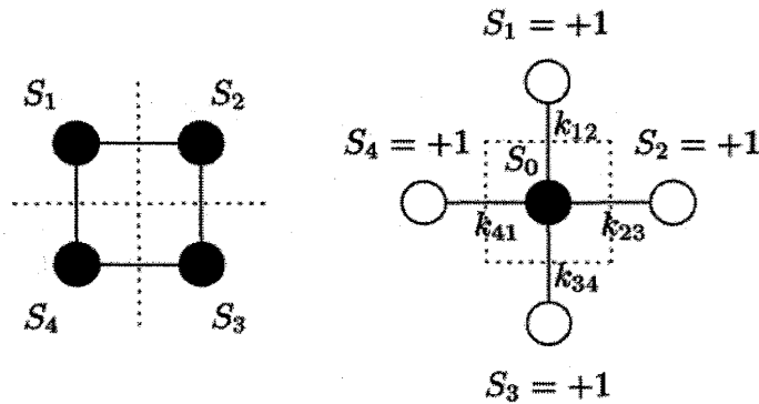
図 5: 4本のボンドを持つ単純な正方格子. 黒丸の部分が和を取るスピンを表す.
