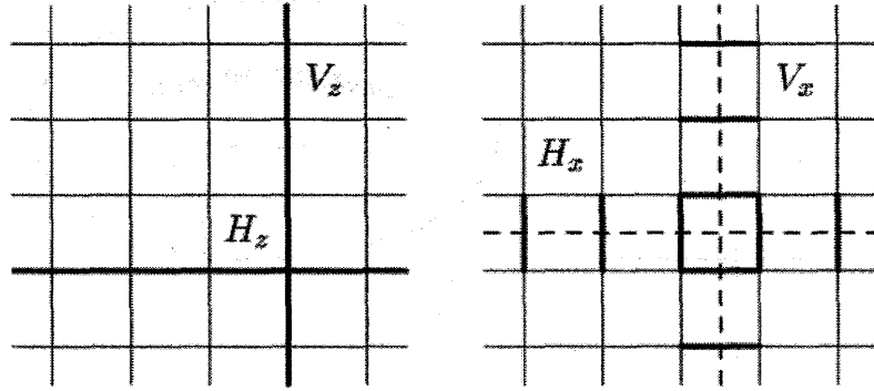
図 40: 符号化演算子 H_i と V_i ( i = x, z ) の作用のさせ方.
