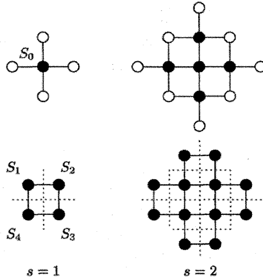
図 29: 正方格子の部分和を多く取るために使用するユニットの例. 上側の図が Z^{(s)} や Z^{*(s)} で表された量を計算するためのユニットであり, 下側がその双対格子であり Z_D を計算する場合に用いる. 黒丸のスピンは部分和を取るものを表しており, 白丸の部分は \{S_i\} = 1 と上向きで固定する条件を課す.
