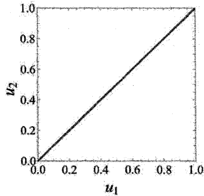
図 14: 西森線上のレプリカ数 2 における \pm J Ising 模型の相対 Boltzmann 因子の振る舞い. ランダムさが ない場合と同様に双対変換前のものと後のものでは完全に一致する.
