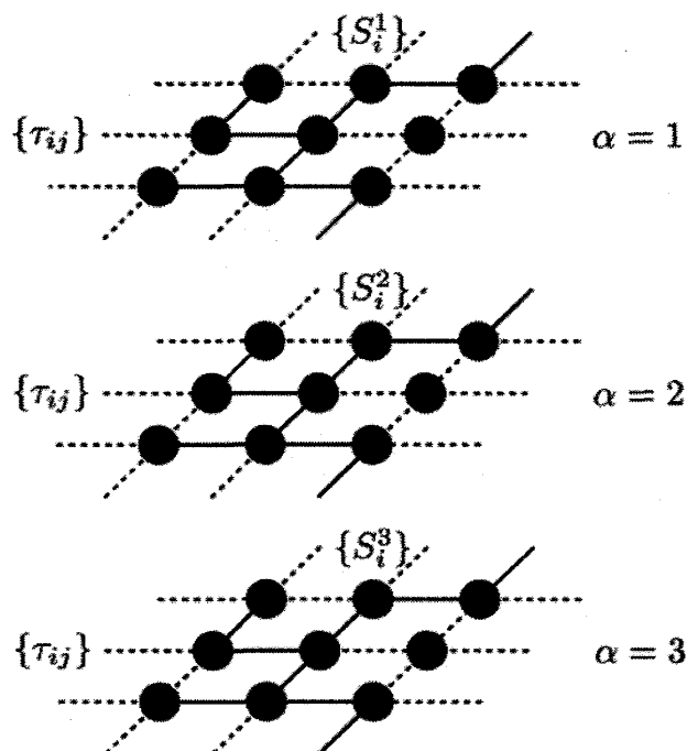
図 4: \pm J Ising 模型のレプリカ法による有効スピン模型. 破線が反強磁性相互作用を表し, 実線が強磁性相互作用を表す.
