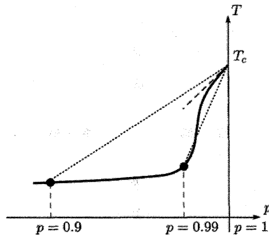
図 33: これまでの結果から類推される相境界の複雑な形状. 破線が双対変換と繰り込みを併用した手法が求めようとしている傾きである.
