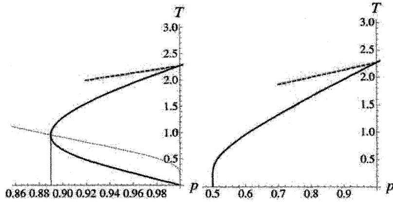
図 24: \pm J Ising 模型 (左図) とボンド希釈型の Ising 模型 (右図) に対する双対変換が予言する相図. 実線が双対変換による相図. 破線が摂動論による解析によって得られたランダムさが少ない領域での相境界を外挿したもの. \pm J Ising 模型に対して西森線を点線で表した. 垂直な直線は数値計算等の結果により期待されている垂直な (もしくはにわかにリエントラントしている) 相境界を比較のために表している.
