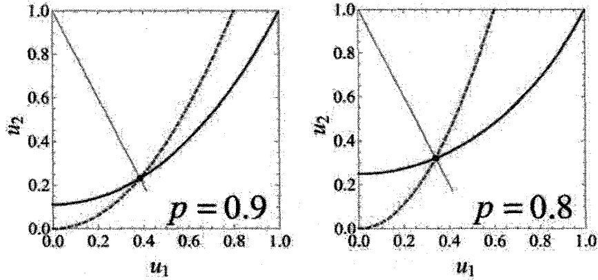
図 13: レプリカ数 2 の場合の有効 \pm J Ising 模型における相対 Boltzmann 因子の振る舞い ( p = 0.9 と p = 0.8 )。実線で表されたのが双対変換前の相対 Boltzmann 因子であり、破線が双対変換後のものを表す。交点として示した点が双対変換の固定点である。直線で表したのが任意の p に対する固定点を連続的に描いたものである。
