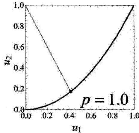
図 12: レプリカ数 2 の場合の有効 \pm J Ising 模型のランダムさが無い場合の相対 Boltzmann 因子の振る舞い. 双対変換前と後で完全に一致する. (図 13 と比較するとよい.) 直線は固定点の集合を表す.
