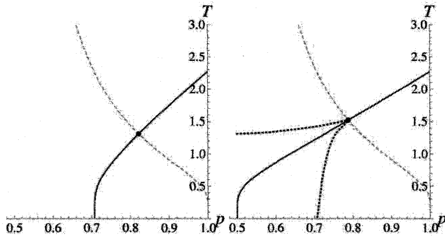
図 11: レプリカ数 1 及び 2 の場合に対する双対変換によって得られる相境界. 破線が西森線を表す. 西森線上の点が多重臨界点を表している. 詳しくは後述するが, 西森線の条件をはずして相境界全体を描く事もできる. 左図で太い曲線はレプリカ数 n=1 に対する有効 \pm J Ising 模型の相境界であり, 右の図の太い曲線は n=2 の場合を表す. 但し n=2 の場合は西森線から上の部分だけで厳密解と一致しており, 下の部分では一致しない. 点線が西森線以下での正しい相境界であり, 単純な相構造をしていない.
