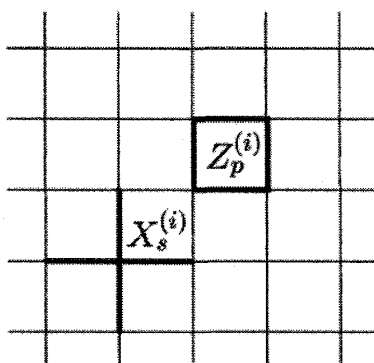
図 38: トーラス符号の構成法. 正方格子上的ボンド上にキュービットを配列する. 縦方向横方向共に周期境界条件をとるため, トーラス符号と呼ぶ.
