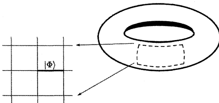
図 38: トーラス符号の構成法. 正方格子上的ボンド上にキュービットを配列する. 縦方向横方向共に周期境界条件をとるため, トーラス符号と呼ぶ.
