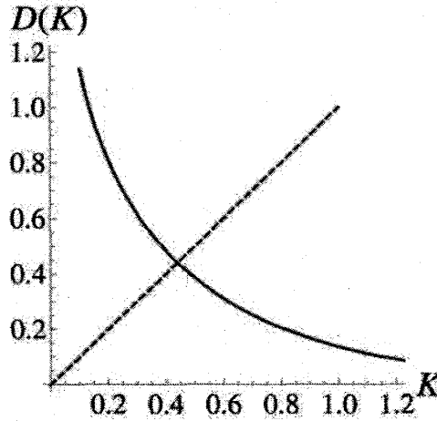
図 9: 逆温度の変換関数 D(K) の様子. 破線は D(K) = K を表す. 交点は逆温度の変換の固定点を表す.
