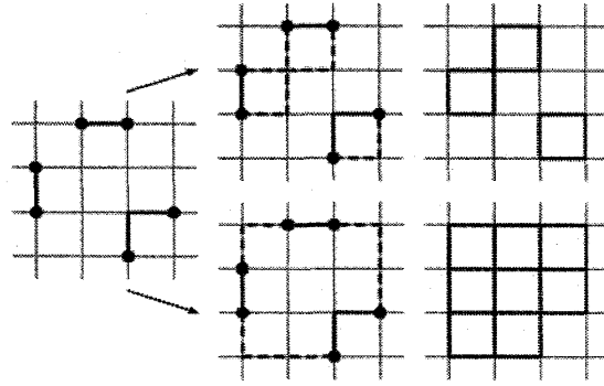
図 41: 反転誤りとその検出. 検査演算の結果 -1 が帰ってきた場合, 黒丸を付しておく.
