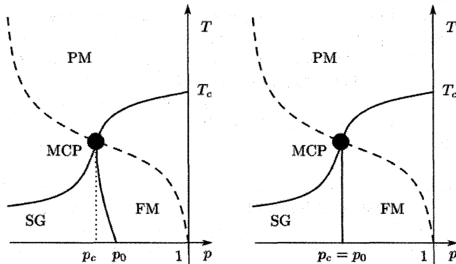
図 1: 考えられている \pm J Ising 模型の相図. 実線が相境界を表す. FM は強磁性相を表し, PM が常磁性相を表す. SG がスピングラス相を表し, 低温にわたって存在する. 実線は相境界である. 破線が西森線を表しており, 多重臨界点は西森線上の点で表されている. 左側はリエントラント転移 ( p_c \neq p_0 ) がある場合. 右側は相境界が西森線以下では垂直 ( p_c = p_0 ) になるとする場合である.
