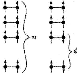
図 10: 相対 Boltzmann 因子の添え字の意味.
