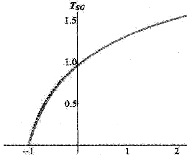
図 34: 破線で示したのが、部分和を用いずに双対変換で得られた転移点のプロット。実線で示されたものが部分和を用いた結果である。非常に小さい幅ではあるが、転移点に変化している様子が伺える。しかしながら n = -1 では絶対零度をどちらの場合も示す。
