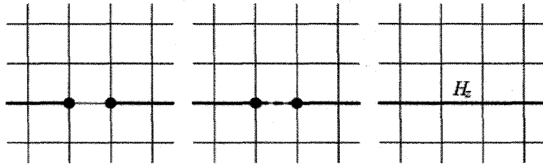
図 43: 周期境界に渡って繋がった誤りが生じた場合の検査演算結果。(真ん中) 最短距離で結ぶ推定法による修正演算。(右側) その修正演算によってもたらされる量子状態への作用。
