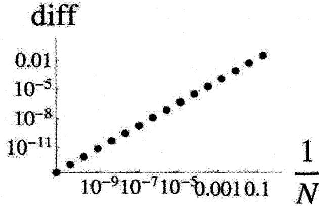
図 30: 厳密解からのずれと繰り返り込みで使用するユニット内のボンド数との関係. 両対数プロットで直線に乗る事がわかる.
