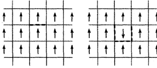
図 44: 誤り（相互作用の分布）と修正演算（スピンの向き反転）の対応．破線が \sigma_z の作用している部分を表す．
