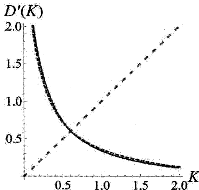
図 23: D'(K) (実線による曲線) とその逆関数 D'^{-1}(K) (破線による曲線) の振る舞い. 点線による直線は D'(K) = K を表す.
