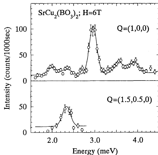
図4：6T磁場中の冷中性子非弾性散乱実験結果 ( k_f=1.55\text{\AA}^{-1} )。 Q=(1,0,0) , (1.5,0.5,0) におけるZeeman分裂した第一トリプレット励起。
