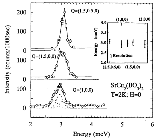
図3：ゼロ磁場中冷中性子非弾性散乱実験結果 ( k_f=1.55\text{\AA}^{-1} )。 Q=(1,0,0) , (1.5,0,0) , (1.5,0.5,0) における第一トリプレット励起のスペクトラ。挿入図：第一トリプレット励起エネルギーの波数依存性。縦棒は single gaussian fit により求められた線幅を示す。
