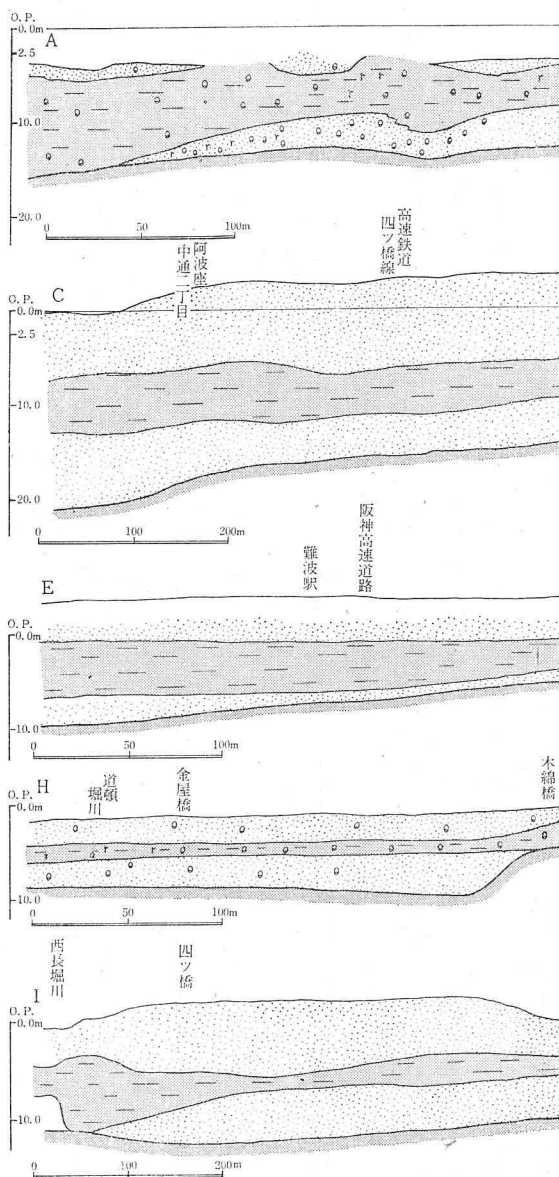
第4図 地質断面図(断面位置は
