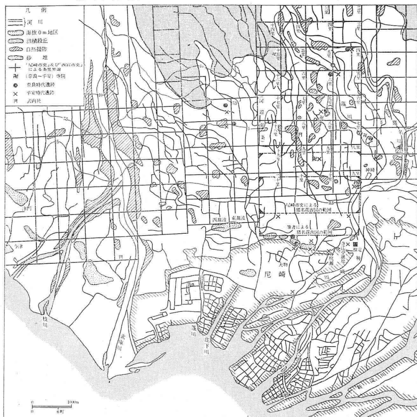
第8図 尼崎付近の地形と条里（地形分類は土地条件図による）
