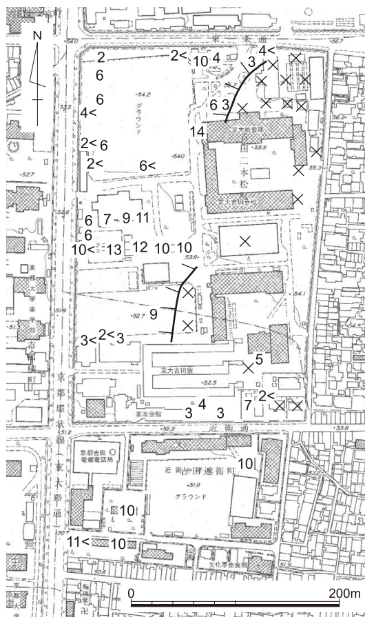
図132 京都大学吉田南構内の黄色砂の層厚 (×10cm) 縮尺1/5000
