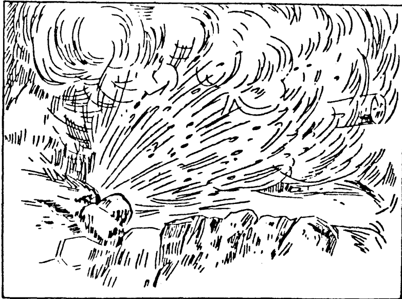
第5図 鬼首ガイザー（論文⑧より）
