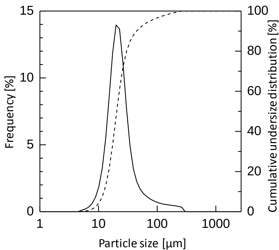
Fig.2 ゼオライトK-CHAの粒子径
