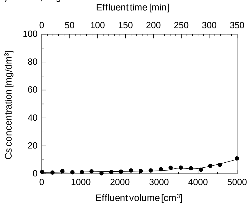
Fig.7 ゼオライトK-CHAの添加量を変えたときの 通液量と装置出口濃度の関係
