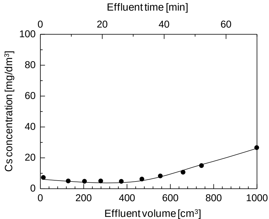
Fig.8 セシウム初濃度を変えたときの 通液量と装置出口濃度の関係
