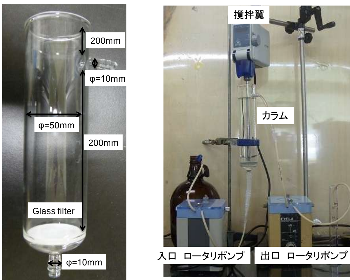
Fig.3 連続通水試験装置
