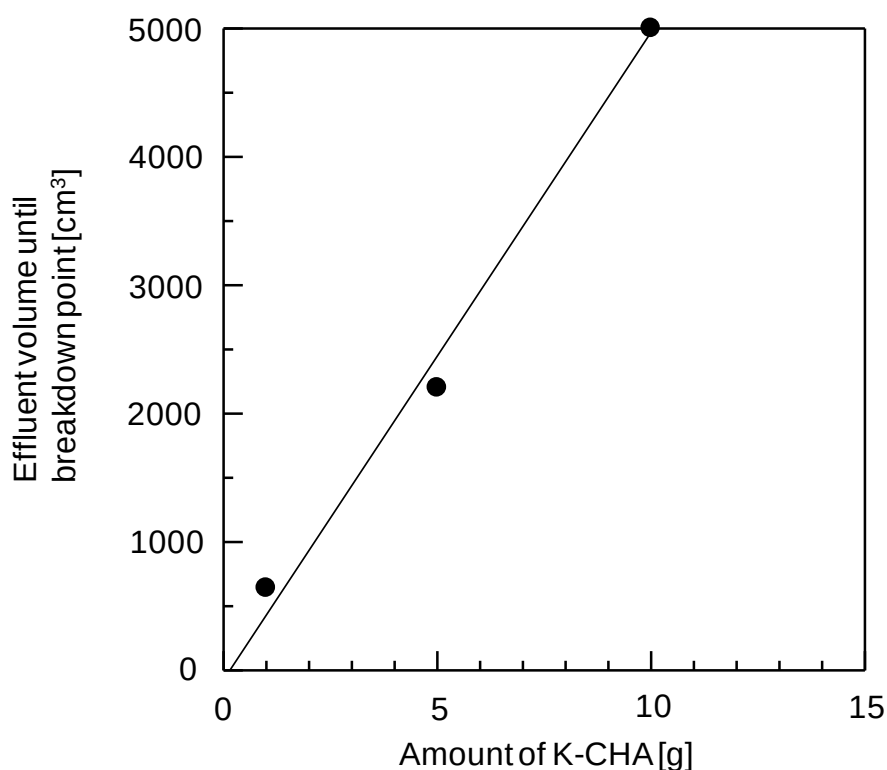
Fig.9 ゼオライトK-CHA添加量と破過点 までの通液量の関係
