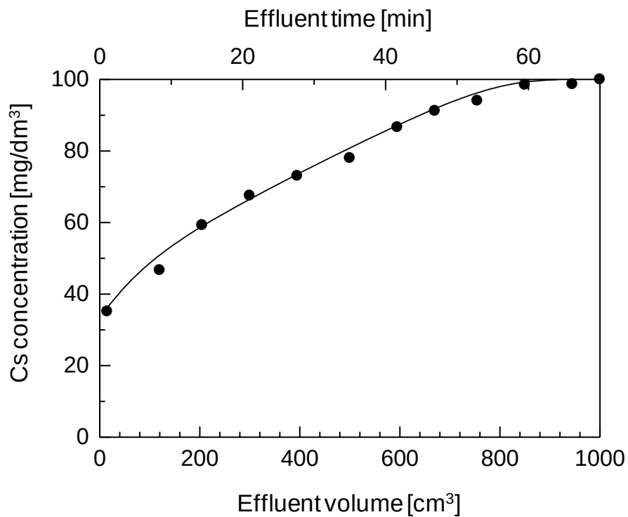
Fig.6 4種のゼオライトを用いたときの 通液量と装置出口濃度の関係
