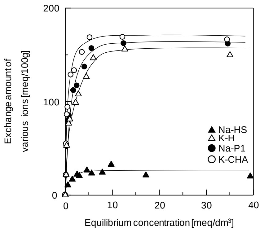
Fig.5 種々のゼオライトによるCs + の吸着等温線
