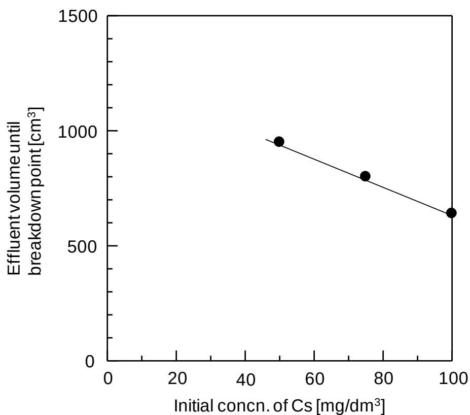
Fig.10 初濃度と破過点までの通液量の関係
