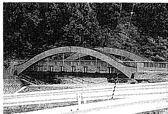
図13 百目石橋（秋田県協和町）
