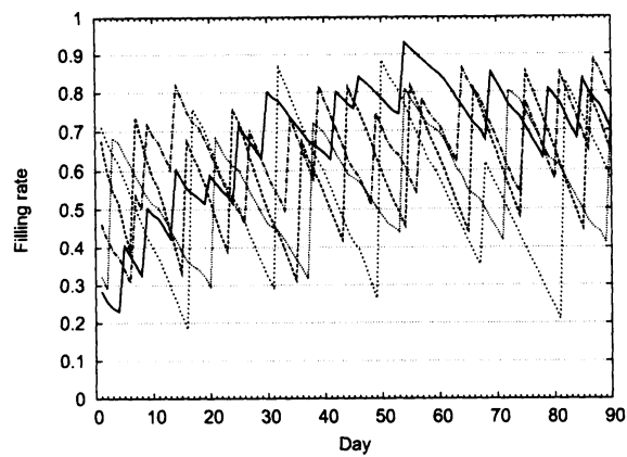
図 7: 先読み期間 60, 実行期間 30
