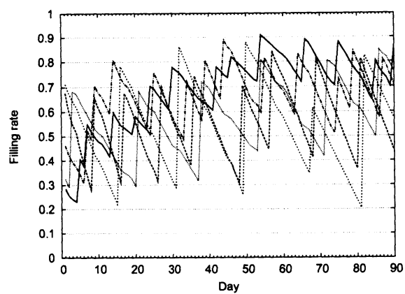
図 6: 動的計画法
