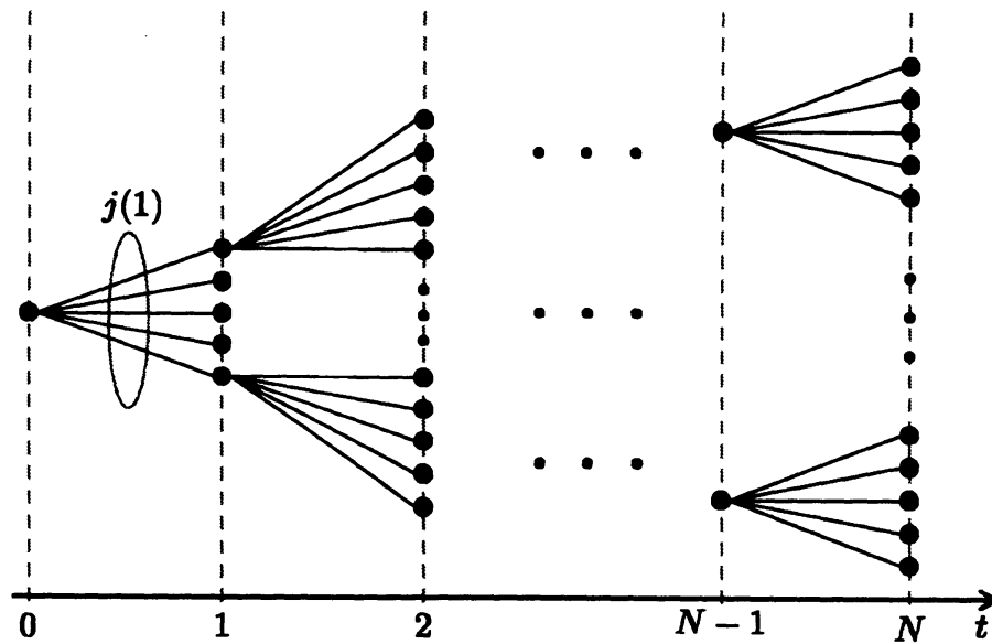
図2: 探索木 (探索木では図の右方向を深さ、上下の広がりをも幅と呼ぶ。)
