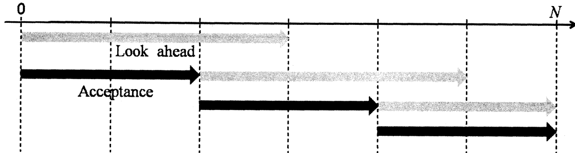
図 3: 近似解法のイメージ
