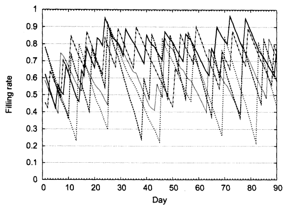
図 12: 動的計画法
