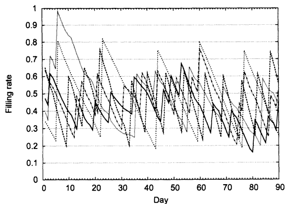
図 9: 動的計画法
