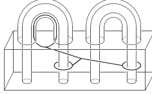
図 1 \Sigma_{2,1} \times [-1, 1] 内のクラスパー.
