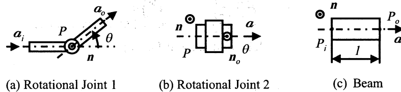
図 4: 機械要素モデル
