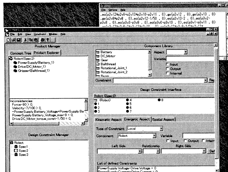
図 3: 初期設計支援システムの概観
