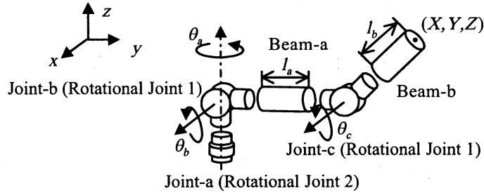
図 5: ロボットアーム
