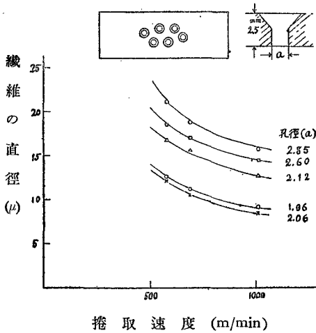
第1圖 捲取速度と繊維の直径との関係
