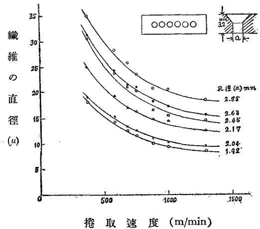
第2圖 捲取速度と繊維の直径との関係
