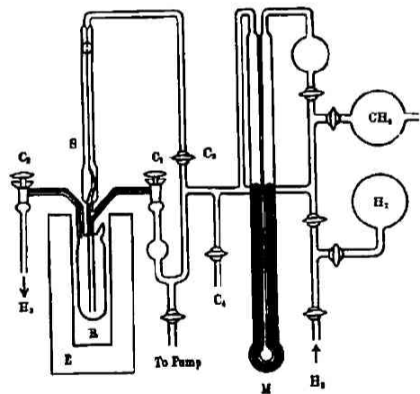
Fig. 1.—Apparatus.
