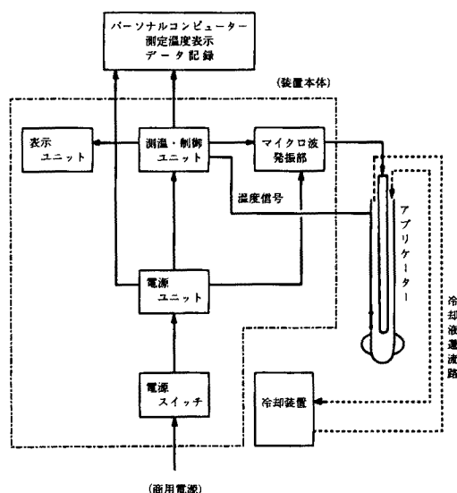
Fig. 1. 温熱療法に用いた装置の説明図
