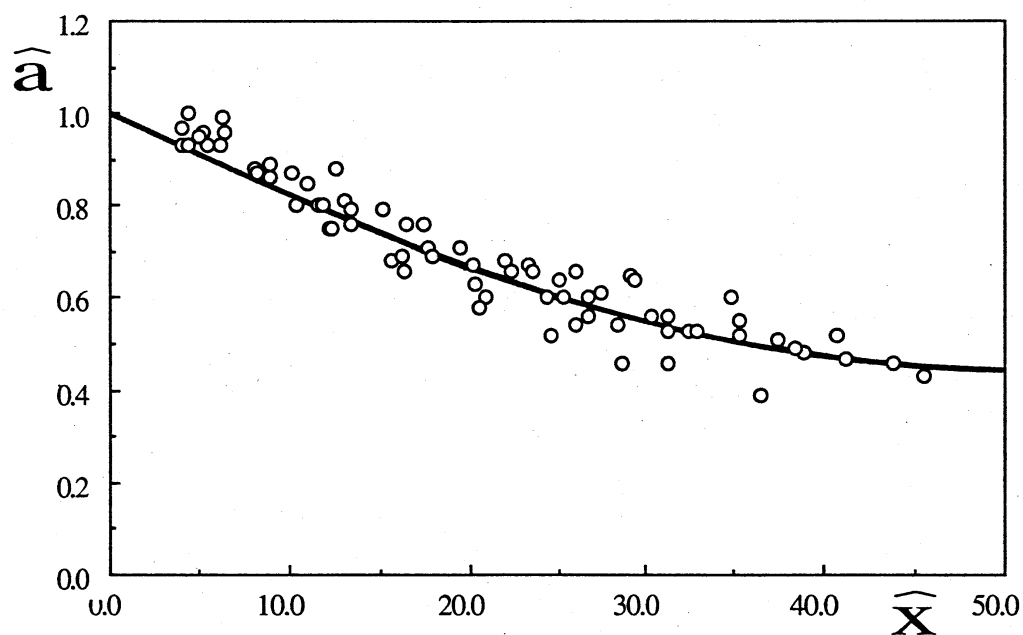
図-3 伝播に伴う内部バルジの振幅の変化
