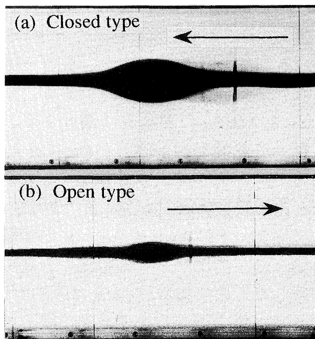
写真-1 内部バルジの伝播 (図中の矢印は伝播方向を示す)
