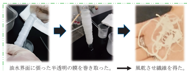
油水界面に張った半透明の膜を巻き取った。→ 風乾させ繊維を得た。
