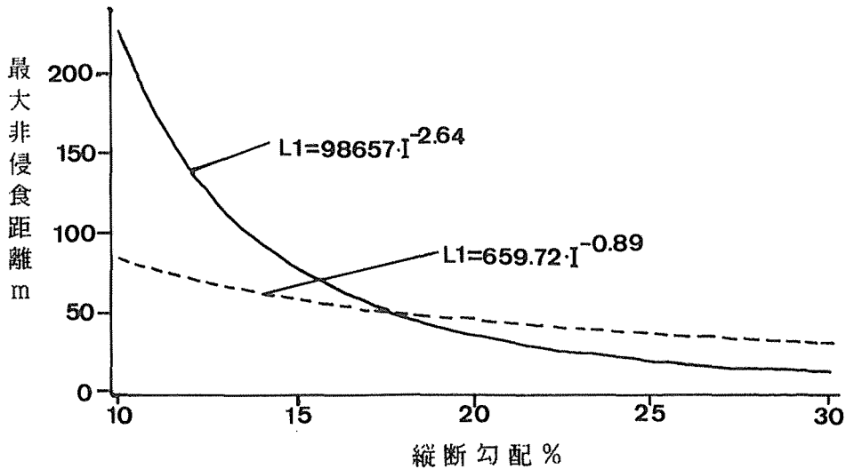
図1 縦断勾配 I と最大非侵食距離 L1 の関係
