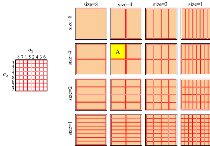
図 10: データ構造
