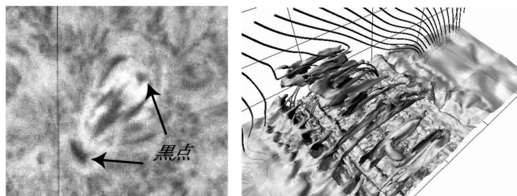
左図: 浮上磁場領域の H\alpha 線像。右図: シミュレーション結果の 3 次元的可視化。細い線は磁力線、グレーは低温高密度のガスの分布を示す。
