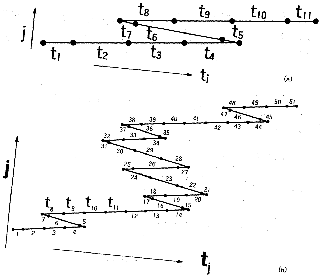
第1図. フラクタル分解:
