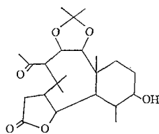
(233)
