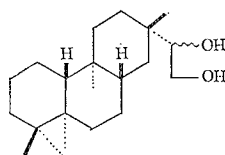
(75)
