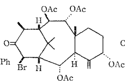
(236)
