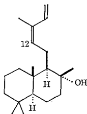
(107)
