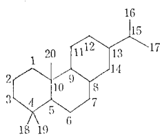
Abietane
