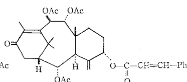
(237)
