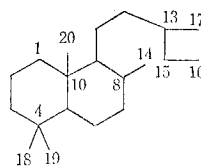
Labdane
