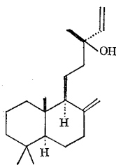
(113)
