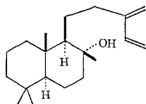
(102)
