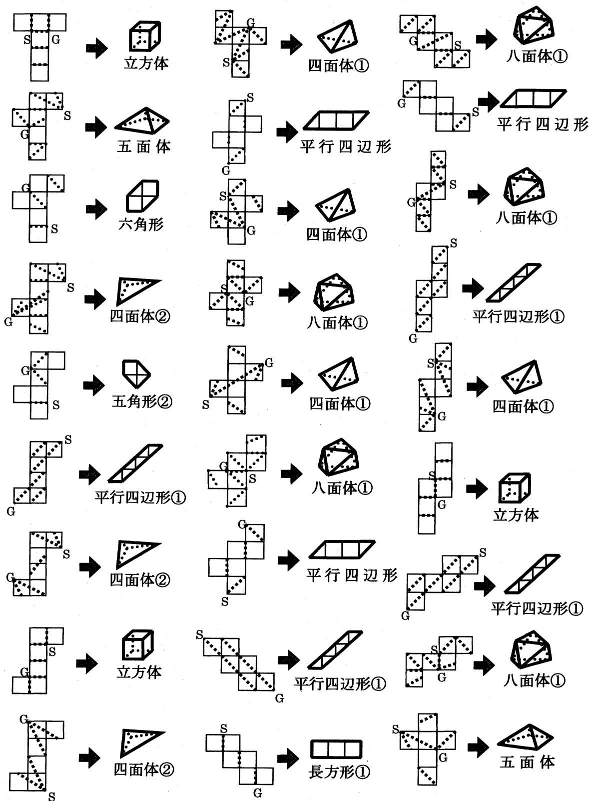
図1 ジッパー再折り凸多面体 (立方体)
