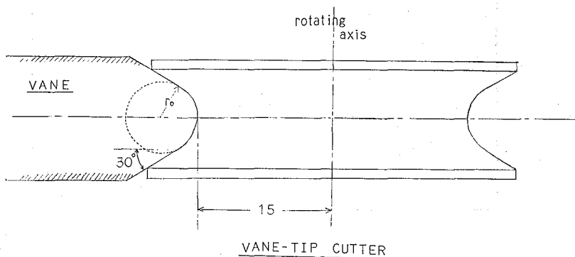
Fig. 5. Vanetip cutter
