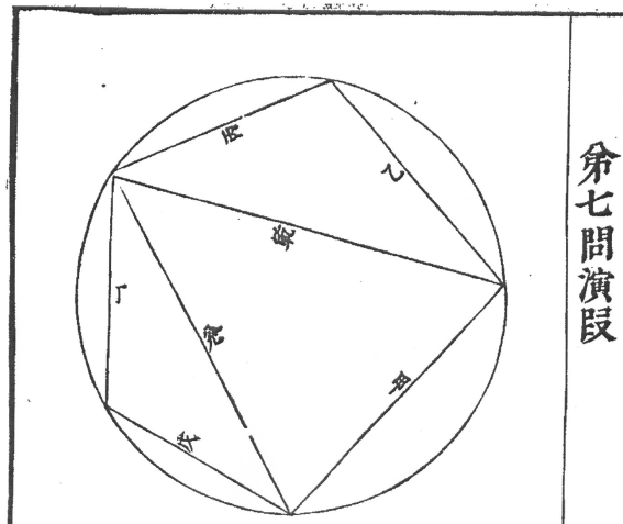
図 1: 「算法發揮」第 7 問
