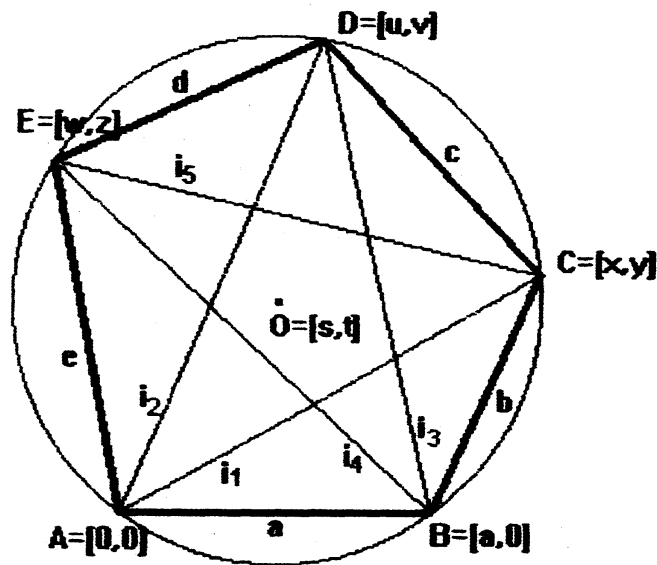
図 2: Pech[4] による定式化
