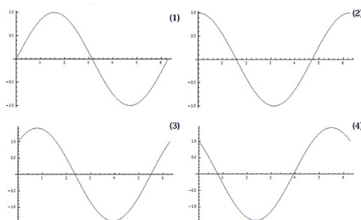
図 8: 連立微分方程式の解のグラフ
