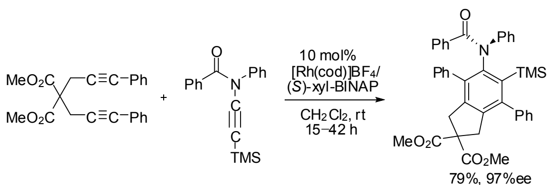
Scheme 28.
