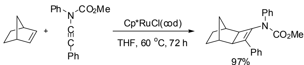
Scheme 30.
