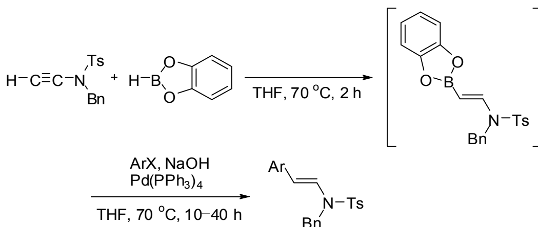
Scheme 23.
