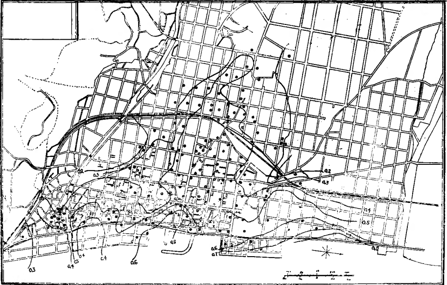
第4圖 別府温泉 \text{HCO}_3^- 變化分布圖 1946年測定値と1927年測定値との差
