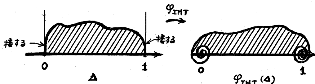
図 2.1 領域 \Delta および Riemann 面 \varphi_{\text{IMT}}(\Delta) の概略図
