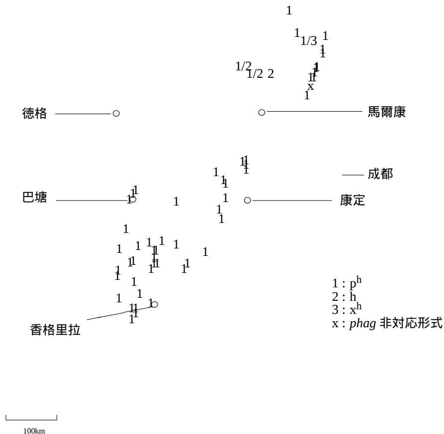
図 2: phag の初頭子音言語地図
