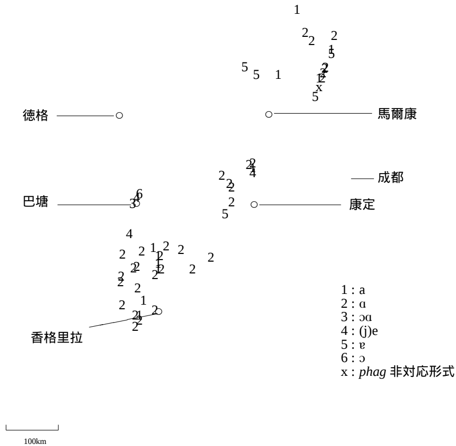
図 3: phag の母音言語地図
