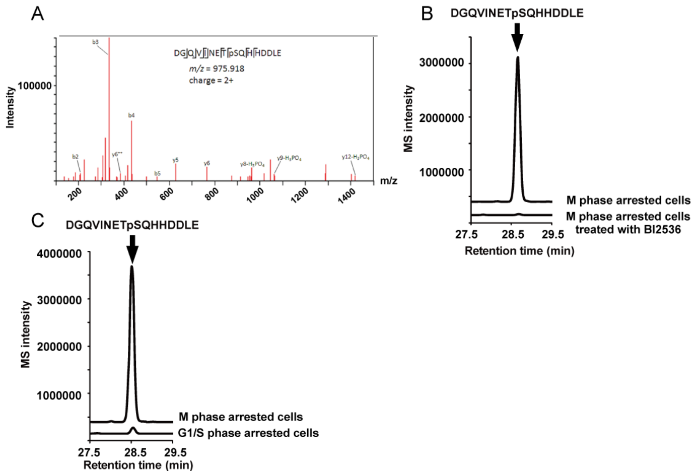
図 16 M 期の細胞内で vimentin の 459 番目のセリンは Plk1 にリン酸化される (A)M 期の細胞をリン酸化プロテオーム解析した結果得られた annotated MS/MS spectra を示している。 (B)(A) の annotated MS/MS spectra から抽出した DGQVINETpSQHHDDLE の ion current chromatogram を示している。 (C)S 期の細胞と M 期の細胞から得られた DGQVINETpSQHHDDLE の ion current chromatogram を示している。
