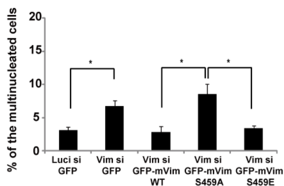
図 28 vimentin の 459 番目のセリンのリン酸化によって細胞質分裂が制御される siRNA を導入した HeLa 細胞に表記のベクターをトランスフェクション後、hoechst によって核を染色した。この細胞のうち、多核化した細胞の割合を求めた。さらにダネット多重比較検定と t 検定を行った。* P < 0.05
