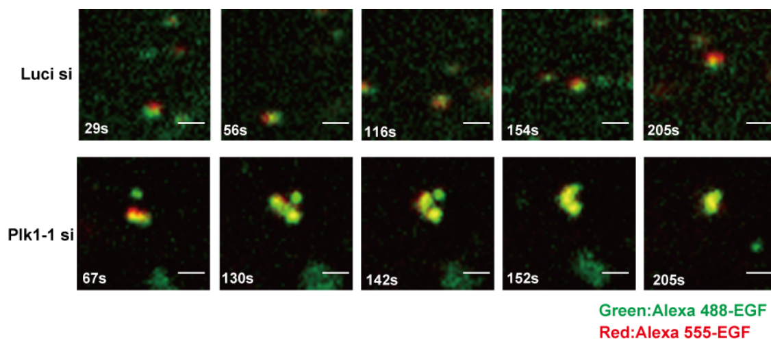
図 10 Plk1 は M 期において初期エンドソームの膜融合を阻害している HeLa 細胞に siRNA を導入後、M 期に同調させ、Alexa555-EGF と Alexa647-EGF を取り込ませて 1 秒間隔でタイムラプス観察を行った。スケールバーは 1μm を示している。
