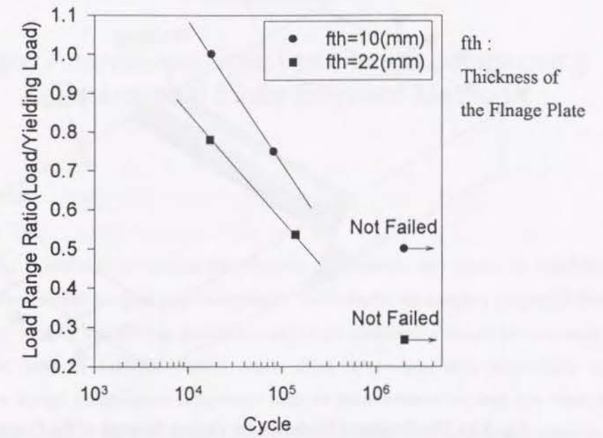
Fig. 4.31 S-N Diagram (1)
