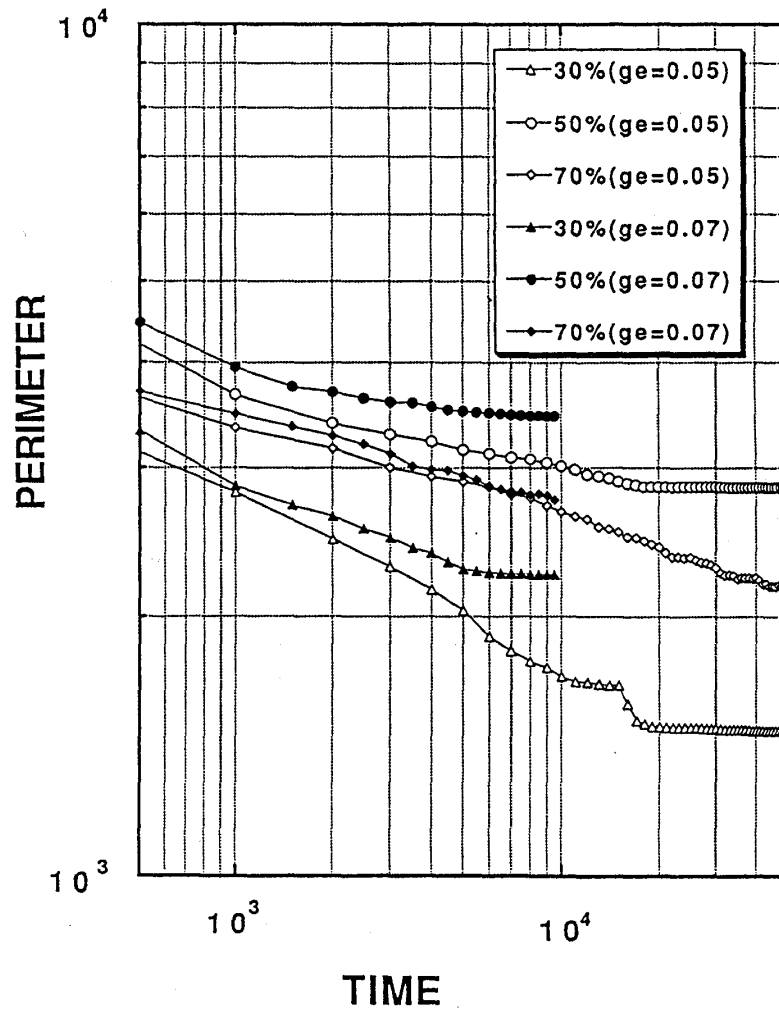
図4, 全体の interface の長さを図示している。 g_e は無次元した \mu_1 である。
