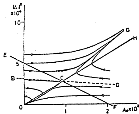
第1図 平均流ゆがみと主擾乱振幅の関係
