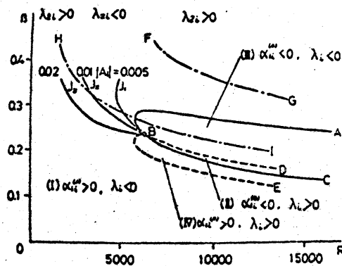
図3 有限擾乱の安定線図
