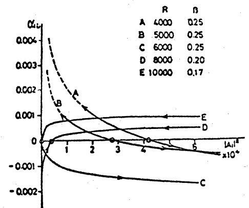
第2図 擾乱振幅と減衰率の関係
