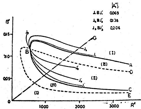
図1 有限攪乱の安定線図
