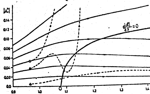
図3 攪乱の主流方向の発達
