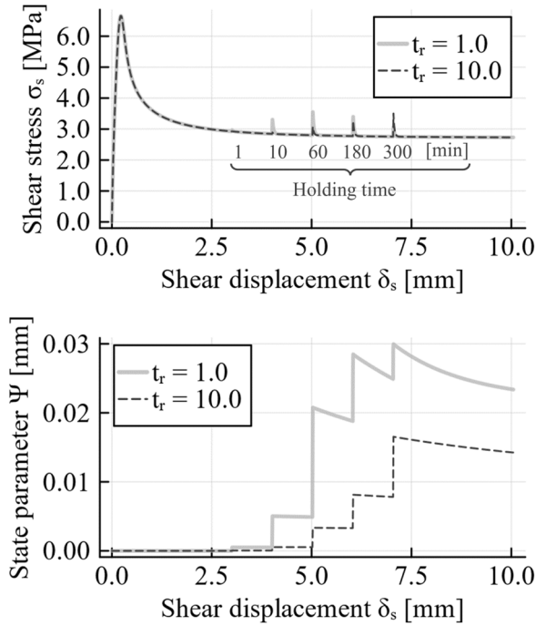
図-10 せん断変位—せん断力—状態変数 \Psi の関係 (パラメータ t_{\text{ref}} に関する感度分析)
