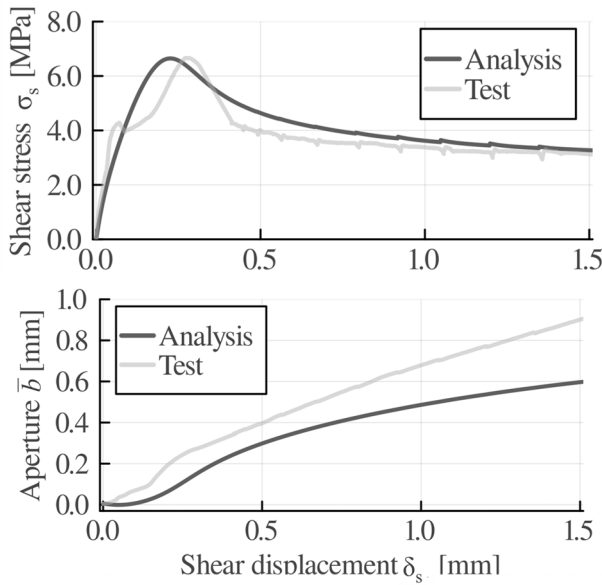
図-8 セン断変位—せん断力—開口幅の関係
