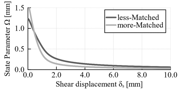
図-5 状態変数 \Omega の変化(解析値)
