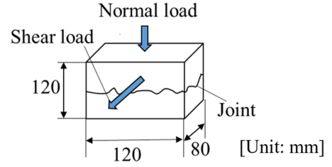
図-7 せん断試験で用いられた不連続面を持つ供試体の概要 24)
