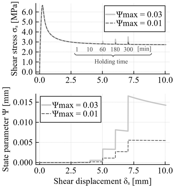
図-11 せん断変位—せん断力—状態変数 \Psi の関係 (パラメータ \Psi_{\max} に関する感度分析)
