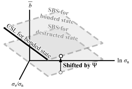
図-6 固着により拡大した状態境界面の概念図
