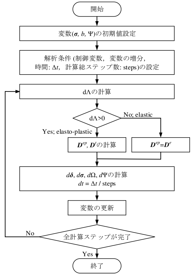
付録 B 図-1 要素解析の計算アルゴリズム
