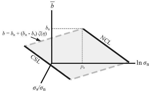
付録A図-1 NCLとCSLの概念図
