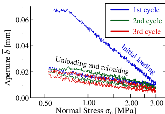
図-1 典型的な岩石不連続面の圧縮挙動 24)
