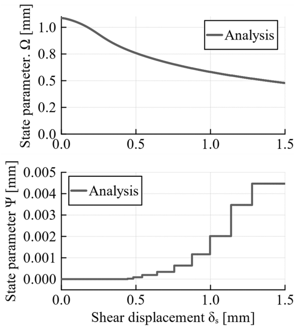
図-9 状態変数 \Omega および \Psi の変化（解析値）
