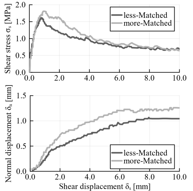
図-3 せん断変位—せん断力—垂直変位関係 16)
