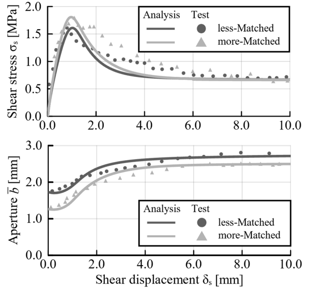
図-4 せん断変位—せん断力—開口幅の関係
