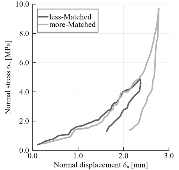
図-2 せん断前の圧縮試験結果 16)
