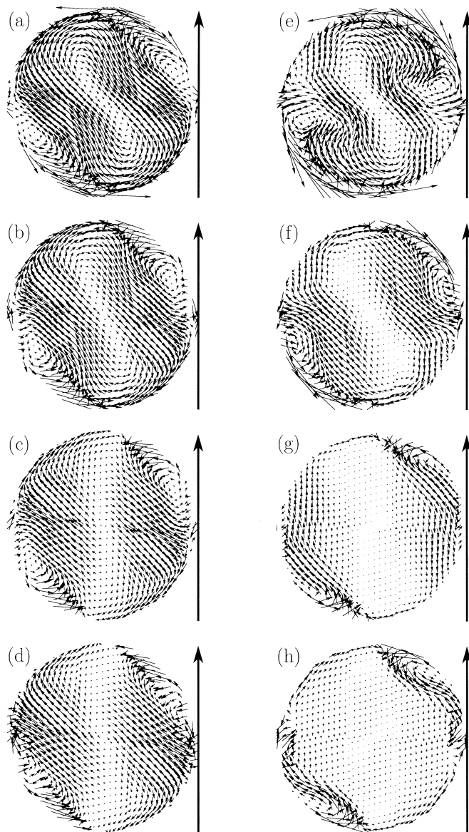
図 6: 赤道面における時間平均流速場. (a–d) 水, (e–h) CTAC 水溶液. (a, e) Re = 1.01 \times 10^4 , (b, f) Re = 2.03 \times 10^4 , (c, g) Re = 4.01 \times 10^4 , (d, h) Re = 8.02 \times 10^4 . Po = 0.1 . 右の太い矢印は壁面速度 a\Omega_s を表す.
