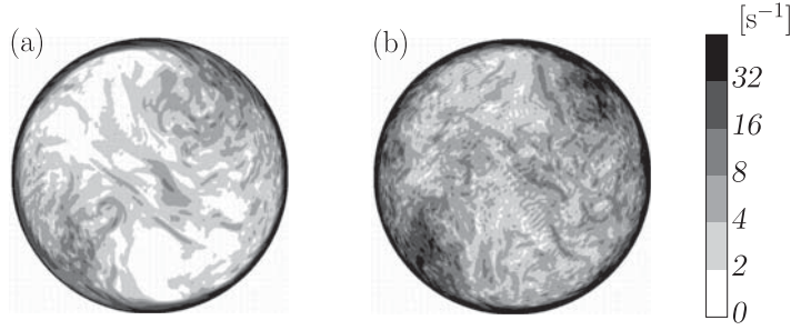
図 5: DNS により求めた乱流中のせん断速度, \dot{\gamma} , の赤道面上の分布. (a) Re = 1 \times 10^4 , (b) Re = 2 \times 10^4 . Po = 0.1 .
