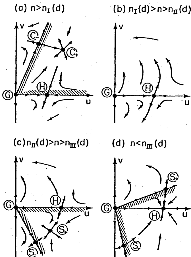
図2 \varepsilon 展開による (u, v) 面での繰り込み群の流れ図。 C_+ がカイラル固定点、 H はハイゼンベルク固定点。 n_I(d) は式(5)で、 n_{II}(d) \simeq 2.20 - 0.57 + O(\varepsilon^2) 、 n_{III}(d) \simeq 2 - \varepsilon + O(\varepsilon^2) で与えられる。
