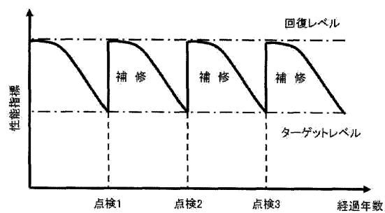
図—2 構造物の性能低下曲線と維持補修の概念
