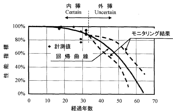
図—1 性能低下曲線のモデル化に関する課題
