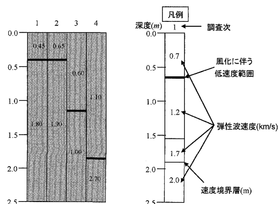
図—4 背面地山のスループット検査結果の一例
