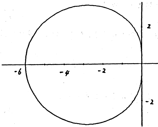
图9. 2段3次Adams-Moulton法
