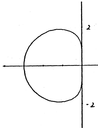
图11. 3段4次Adams-Moulton法
