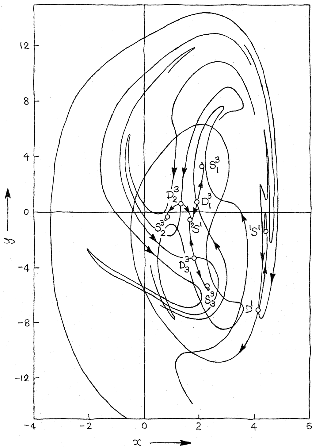
カ7図 \bar{\epsilon}=0.1 , B=18.4 に対する phase diagram
