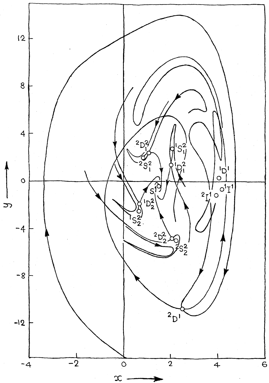
图 6 图 R=0.07 , B=16.1 に対する phase diagram
