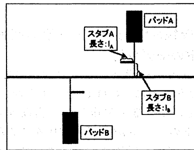
(a) 設計図
