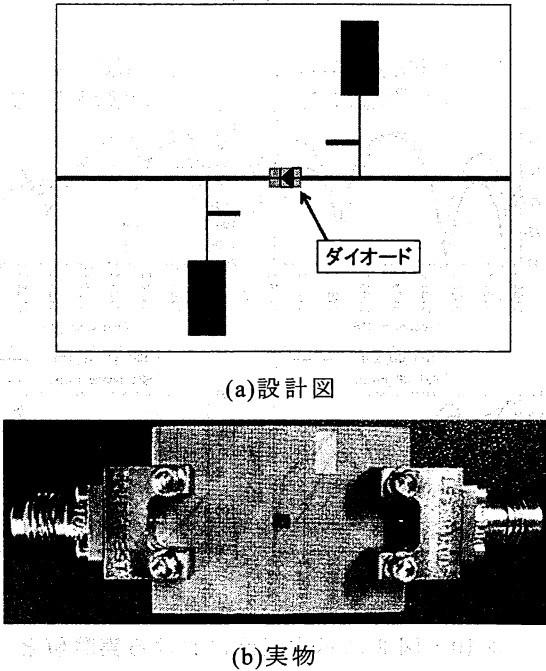
図 11：直列接続型ダイオード特性測定用治具回路
