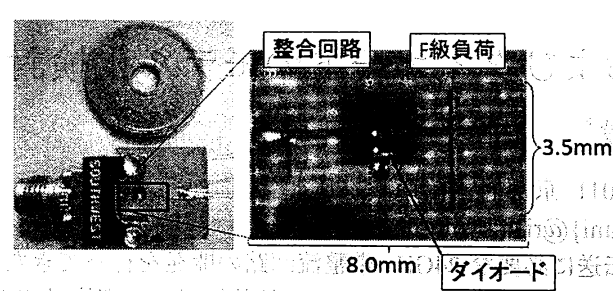
図 2：ダイオード 2 並列 F 級負荷装荷整流回路
