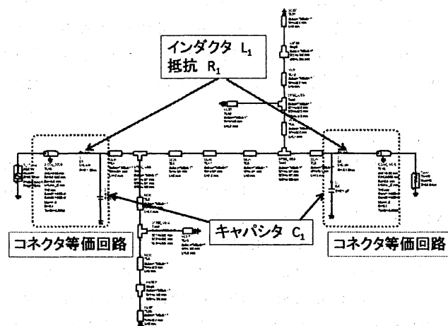
図 9：コネクタ等価回路を含むシミュレーションモデル
