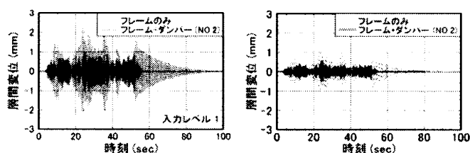
図11 変位の時刻歴応答
