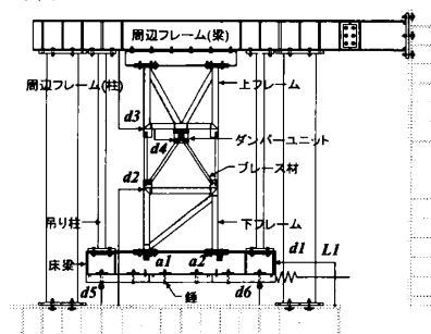
図4 供試体の概要と計測計画
