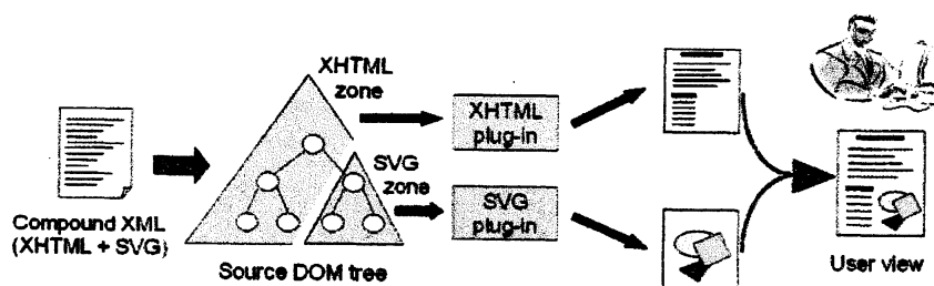
図1 xfy における複合 XML の処理
