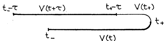
図2. 積分路と行列要素のとり時刻
