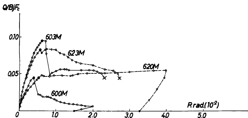
Fig. 5 (d) Load vs. deflection for h/D=6 .
