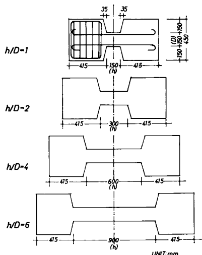
Fig. 1 Test specimen.
