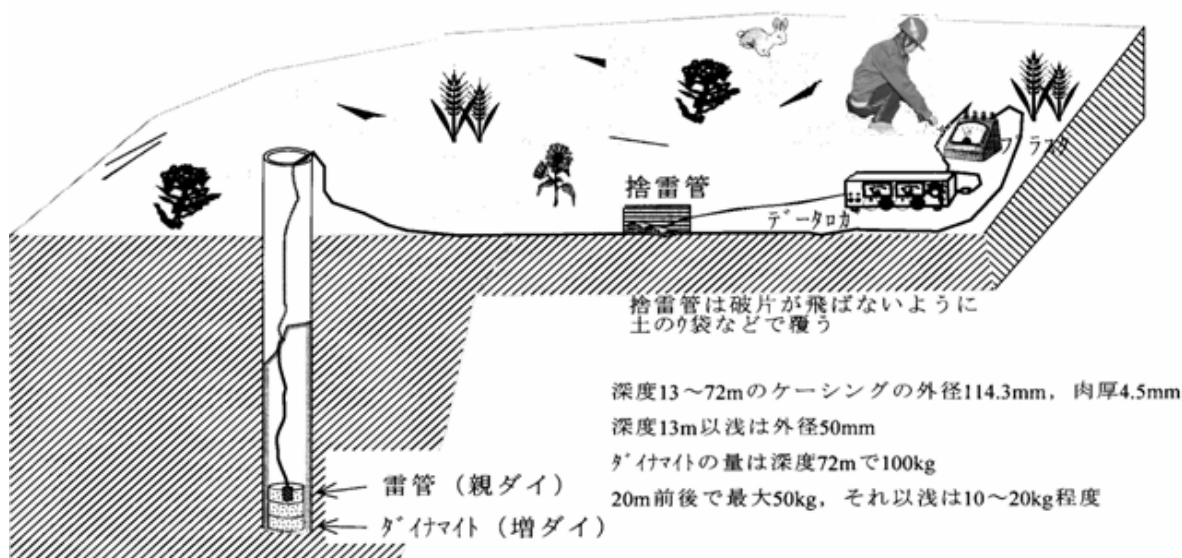
図 3 発破作業の模式図
