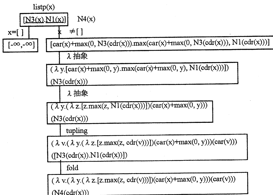
図4 : タプリング( \text{N3}(x) と \text{N1}(x) の同時計算)に対するGPC木
