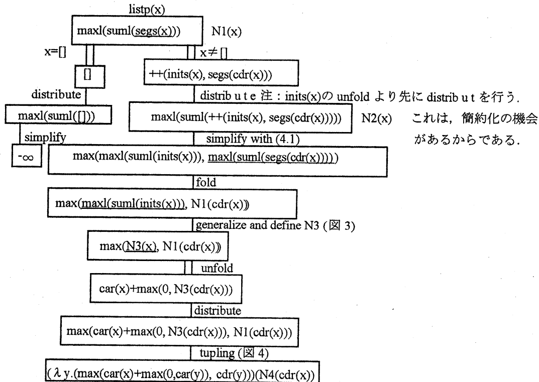
図2 : x がリスト( \text{listp}(x) )である場合の \text{maxl}(\text{suml}(\text{segs}(x))) のGPC木
