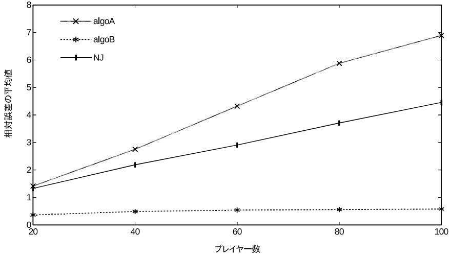
図 11: 一様ランダムな費用関数 c に対する \frac{\|\text{Sh}(\tilde{c}) - \text{Sh}(\tilde{c}')\|_2}{\|\text{Sh}(\tilde{c})\|_2} の平均値.
