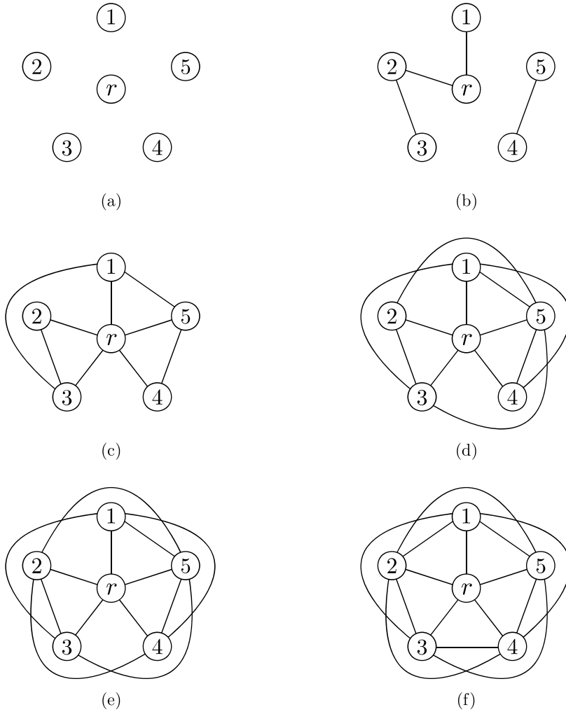
图 8: (a) G'_0 ; (b) G'_1 ; (c) G'_2 ; (d) G'_3 ; (e) G'_4 ; (f) G'_5 .
