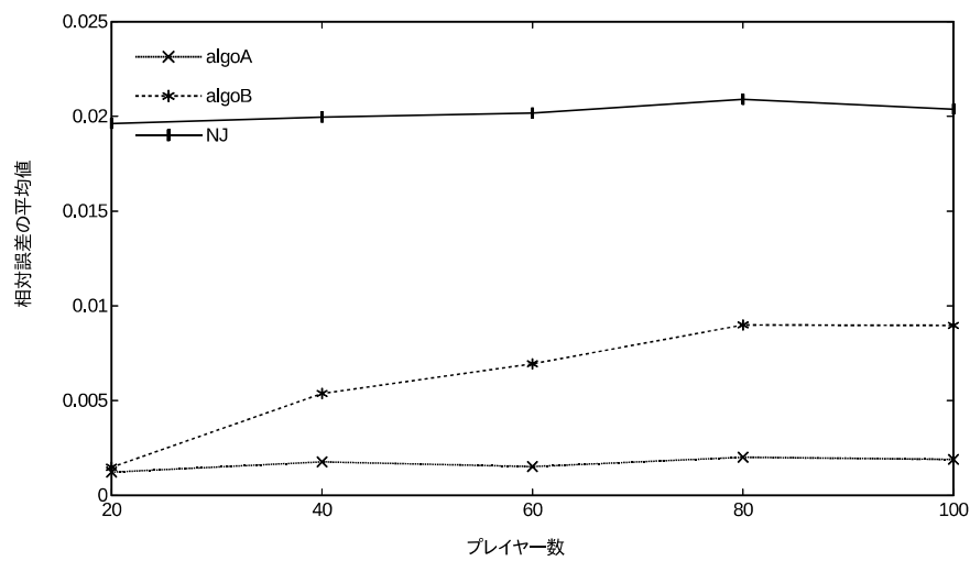
図 13: 木距離を摂動させた費用関数 c に対する \frac{\|c-c'\|_2}{\|c\|_2} の平均値.
