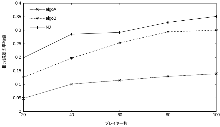
図 12: 2次元ユークリッド距離 c に対する \frac{\|c - c'\|_2}{\|c\|_2} の平均値.
