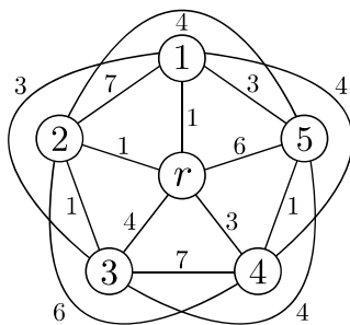
図 3: ネットワーク (K_{N'}, c) .
