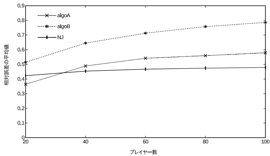
図 14: 一様ランダムな費用関数 c に対する \frac{\|c-c'\|_2}{\|c\|_2} の平均値.
