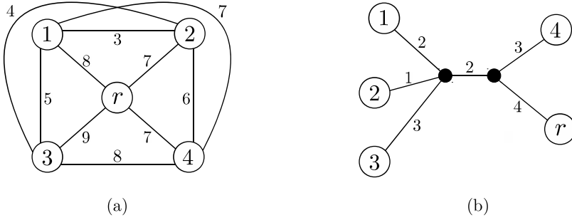
図 5: (a) c が木距離であるネットワーク (K_{N'}, c) ; (b) c を表現する木.
