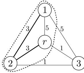
図 2: 部分グラフ K_{S'} と (K_{S'}, c) の最小費用全域木.
