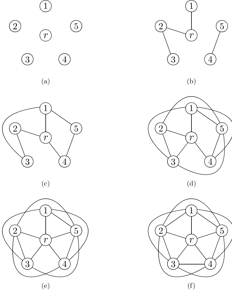
図 6: (a) G(c_0) ; (b) G(c_1) ; (c) G(c_2) ; (d) G(c_3) ; (e) G(c_4) ; (f) G(c_5) . G(c_0), G(c_1), G(c_4), G(c_5) はコーダルであり, G(c_2), G(c_3) はコーダルでない.
