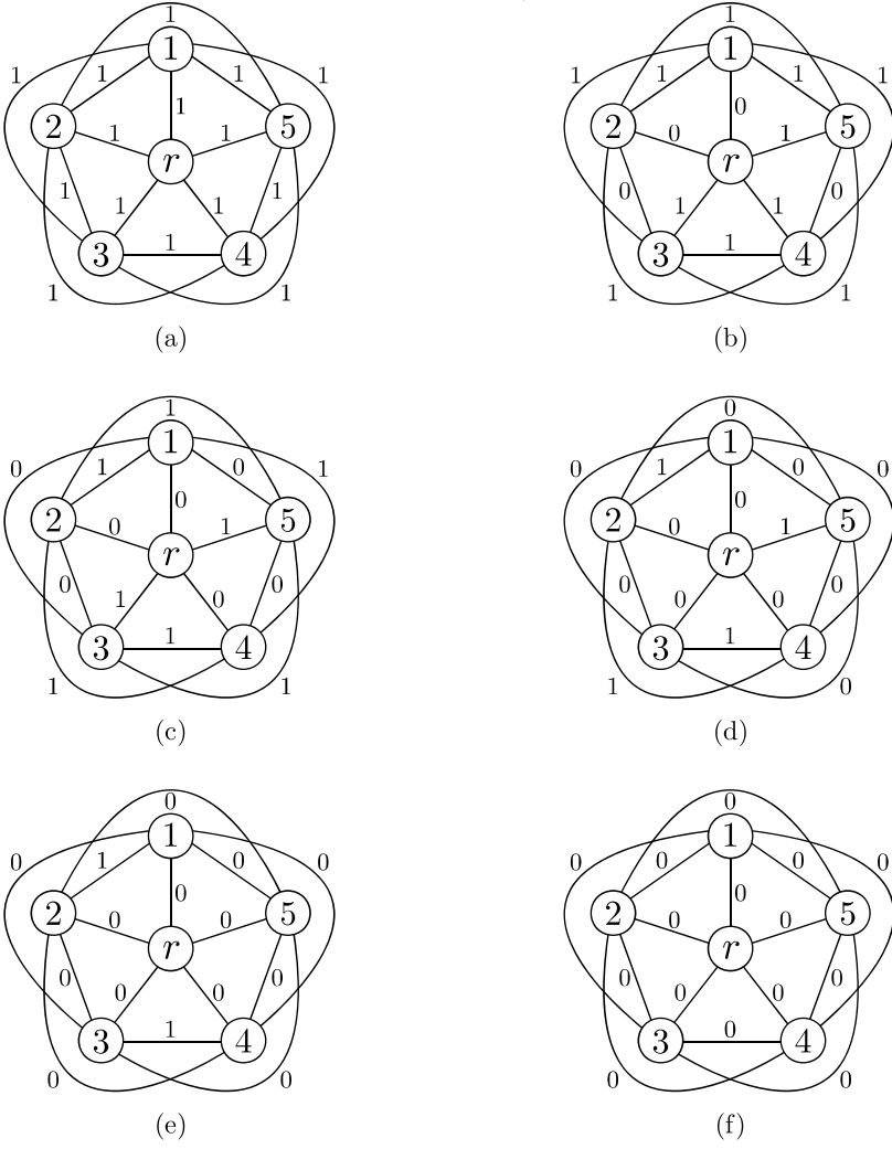
图 4: (a) (K_{N'}, c_0) ; (b) (K_{N'}, c_1) ; (c) (K_{N'}, c_2) ; (d) (K_{N'}, c_3) ; (e) (K_{N'}, c_4) ; (f) (K_{N'}, c_5) .
