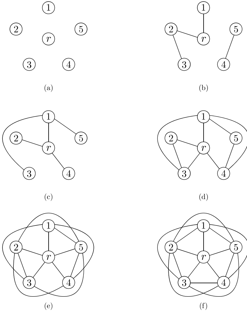
图 7: (a) G'_0 ; (b) G'_1 ; (c) G'_2 ; (d) G'_3 ; (e) G'_4 ; (f) G'_5 .
