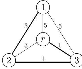
図 1: ネットワーク (K_{N'}, c) と最小費用全域木.
