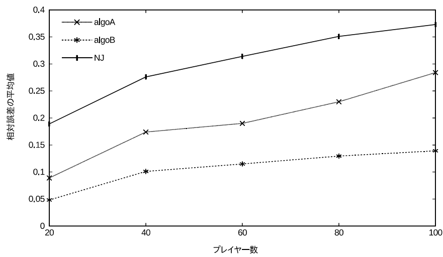
図 9: 2次元ユークリッド距離 c に対する \frac{\|\text{Sh}(\tilde{c}) - \text{Sh}(c^*)\|_2}{\|\text{Sh}(\tilde{c})\|_2} の平均値.
