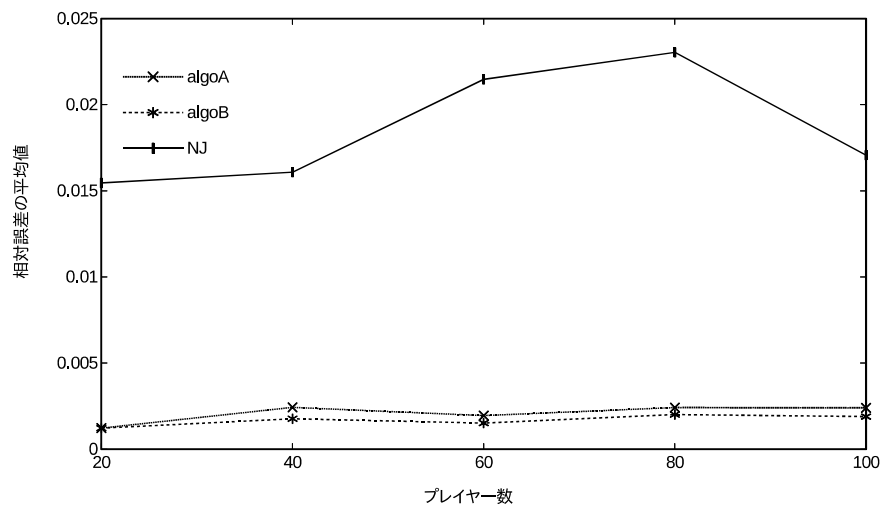
図 10: 木距離を摂動させた費用関数 c に対する \frac{\|\text{Sh}(\tilde{c}) - \text{Sh}(c^*)\|_2}{\|\text{Sh}(\tilde{c})\|_2} の平均値.
