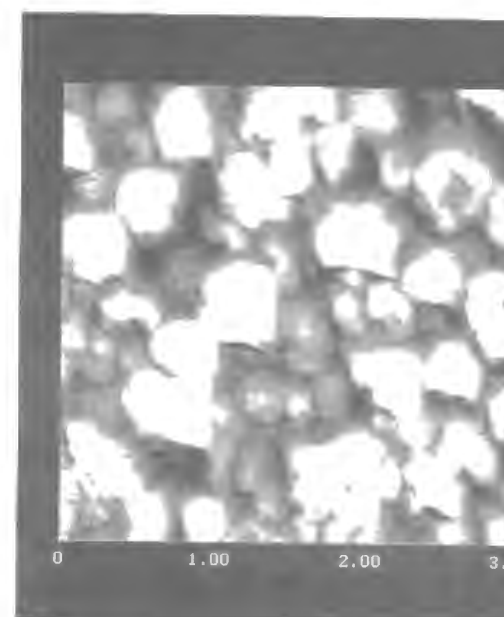
(d) 60 mC cm -2 dissolution
