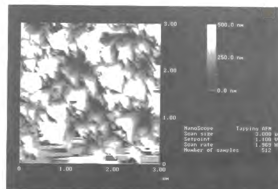
(f) 190 mC cm -2 dissolution
